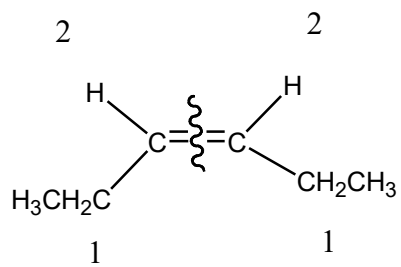
(Z)-3-hexene
